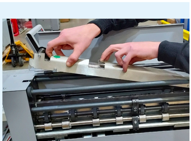
Sacar la tapa de seguridad 'EasyBlade'
