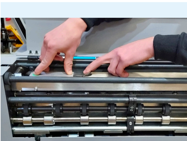
Mecanismo de cambio rápido EasyBlade
